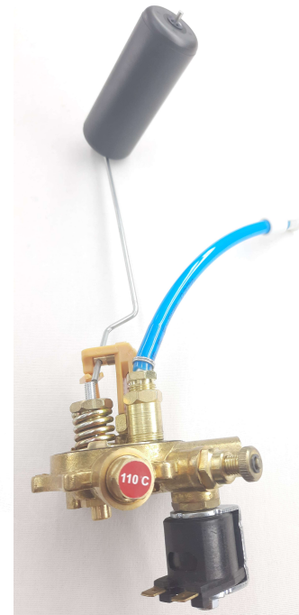
TOROIDAL MULTIVALVE E67R 01
